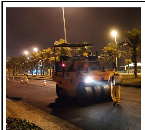
AV. LUCIO COSTA COMPACTAÇÃO (2ª CAMADA)
